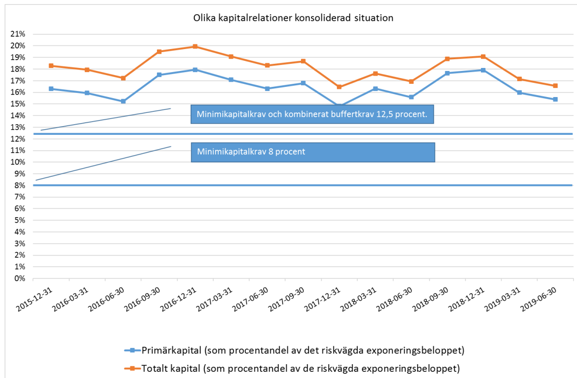
Diagram 1: Olika kapitalrelationer Avanza konsoliderad situation.
